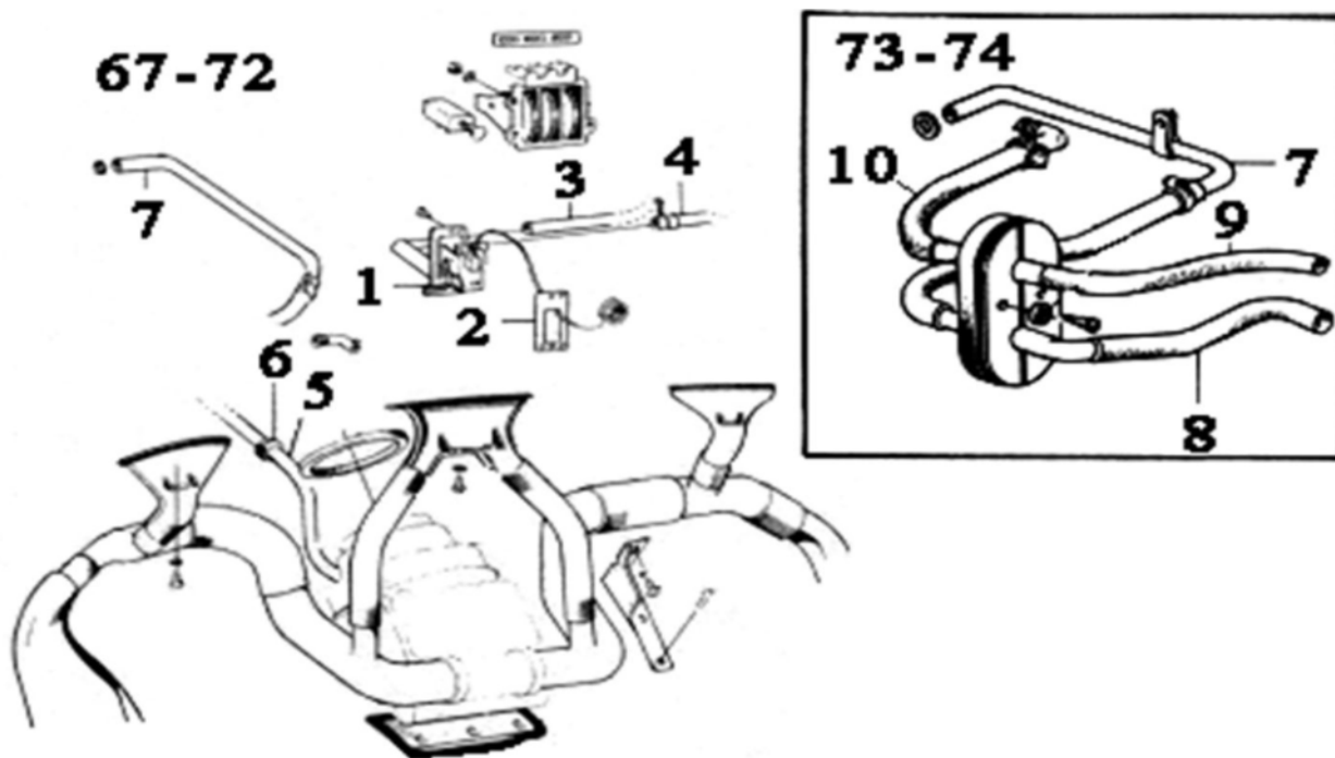
Fig 1: Värmesystem 140
