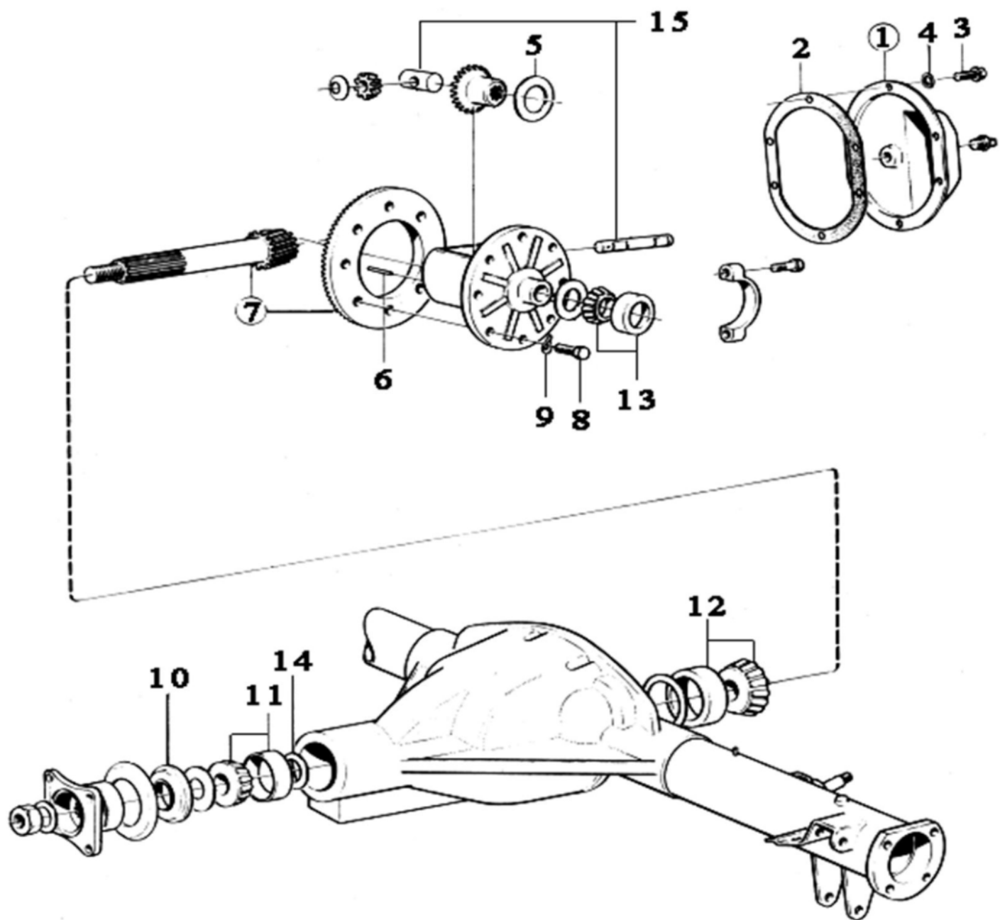
Fig 4: Bakaxel 140 (67-72)
