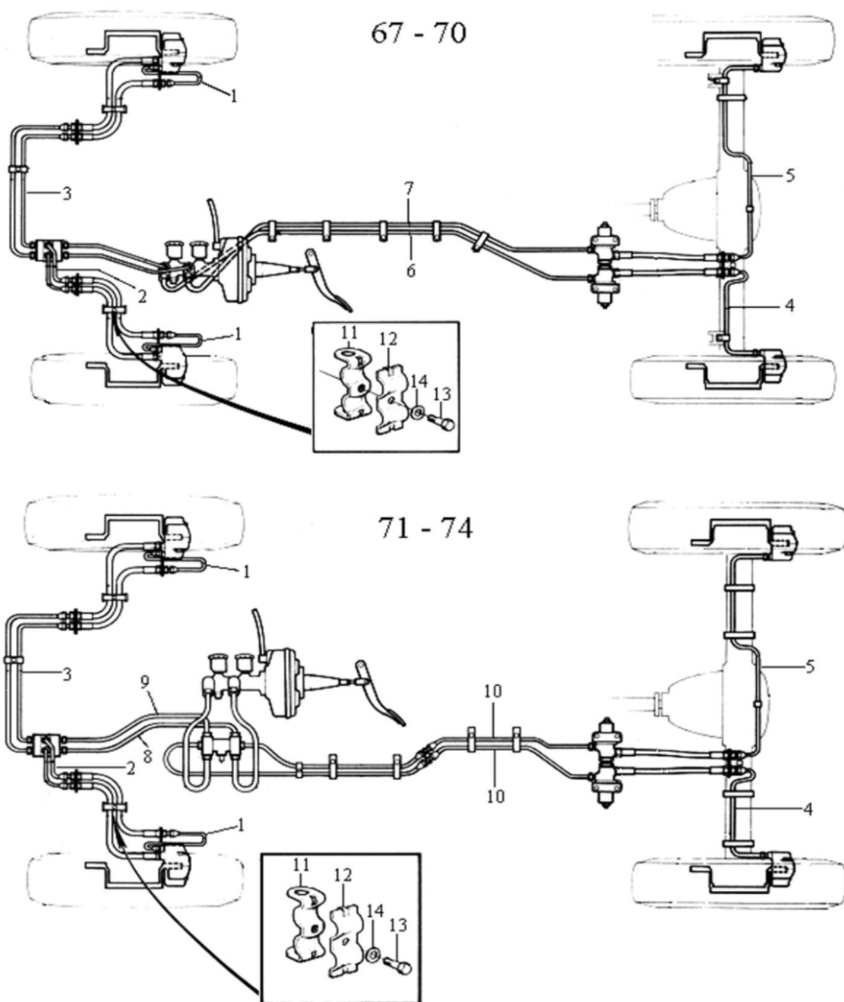
Fig 6: Bromsrör
