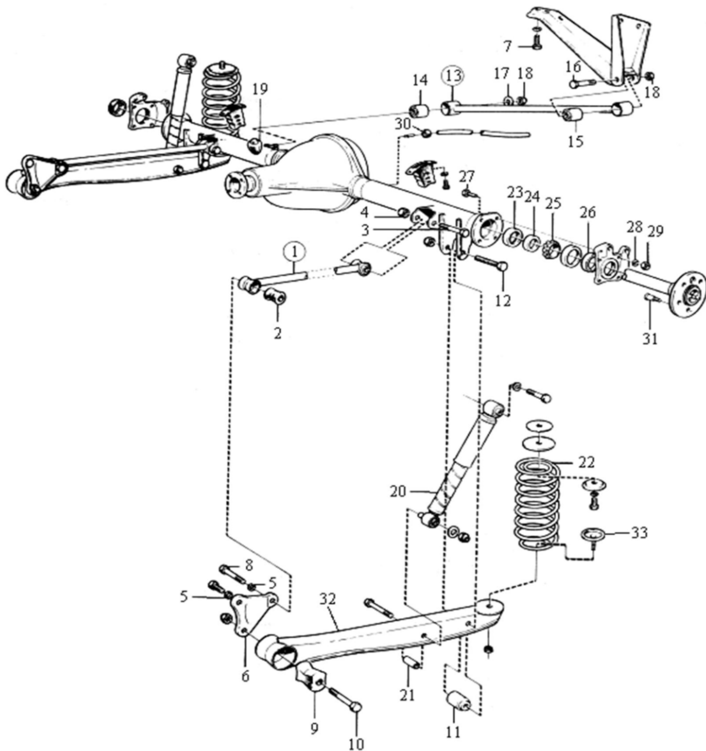
Fig 3: Upphängning bakaxel, 140 (67-72)
