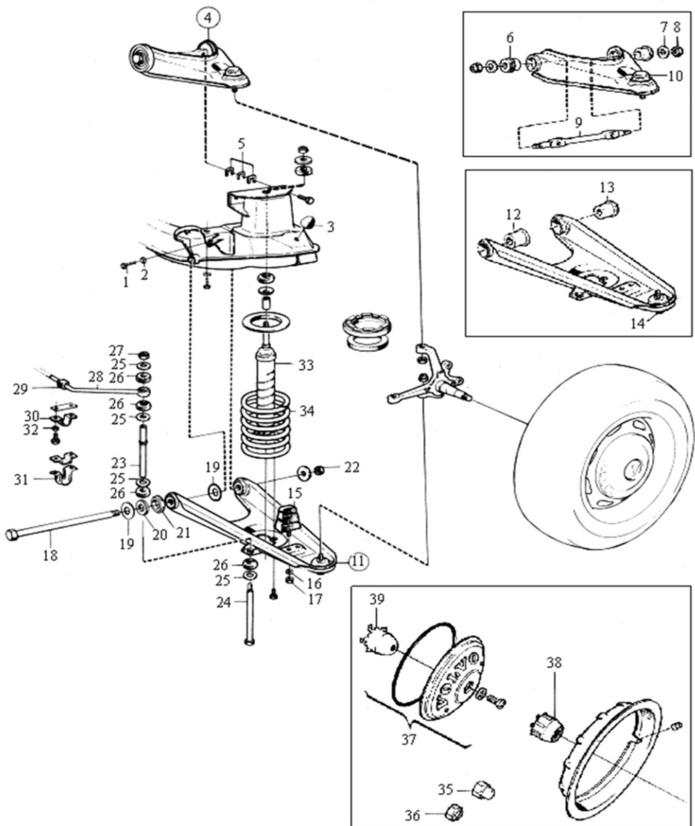
Fig 2: Framvagn 140 (67-72)
